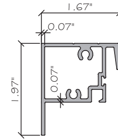
⑤ SASH TOP YY86-43 6063-T5
