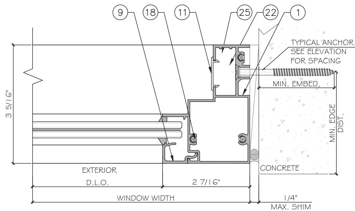
3 D2 DETAIL
