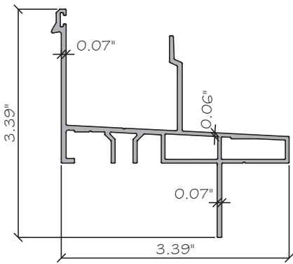
② FRAME SILL YY86-40 6063-T5
