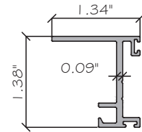
⑦ VENT JAMB YY86-45 6063-T5
