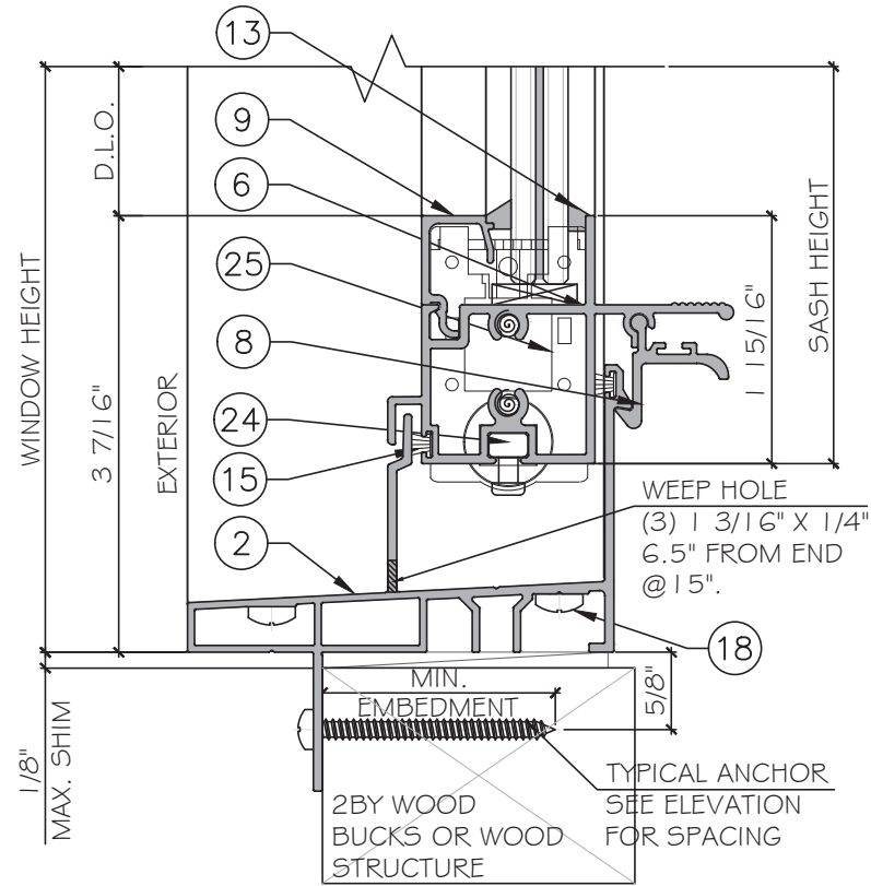
2 D3 DETAIL
