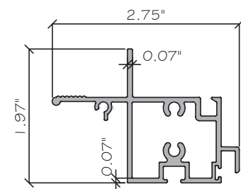
⑥ SASH BOTTOM YY86-44 6063-T5
